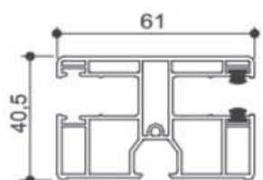
Universele Führungsschiene PVC mini Art. X25052
