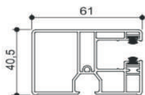
Seitliche Führungsschiene PVC mini Art. X25060
