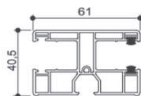
Universele Führungsschiene PVC maxi Art. X91104
