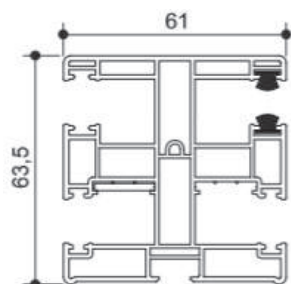
Führungsschiene PVC für Rollläden mit Insektenschutzgitter Art. X25084
